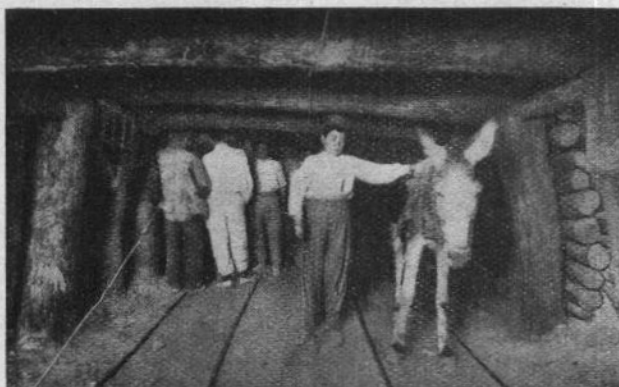
Galería central de transporte. «Coto Menor de Hellín», S. A.
