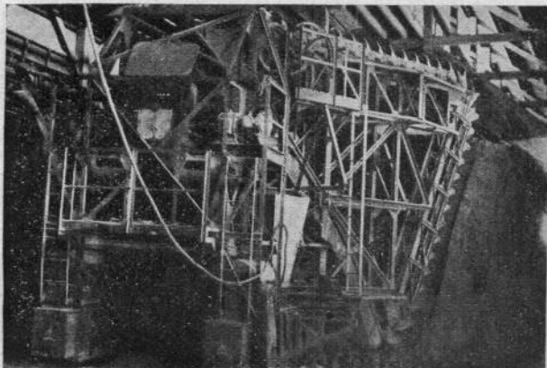
Carro París para arranear, desintegrar y envasar superfosfatos de la Unión Española de Explosivos.
