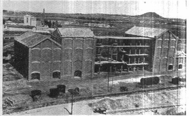
Edificio para el nuevo oleum de la Unión Española de Explosivos.
