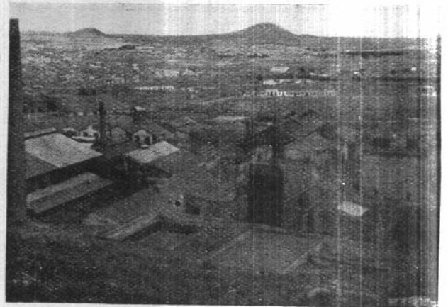
Fundición de Santa Lucía, en Cartagena, de la Sociedad Minero-Metalúrgica de Peñarroya. Vista de conjunto.
